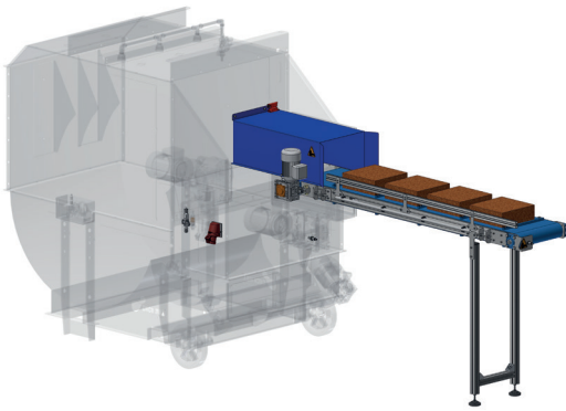
Semi-automatische invoerband Semi- automatic Infeed belt Transportador de alimentación semi-automático
