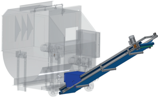
Uitvoerband 2900 mm lang Outfeed belt 2900 mm long Cinta de salida 2900 mm de largo
