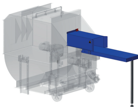
Handmatig invoerplateau Manual infeed tray Bandeja de alimentación manual
