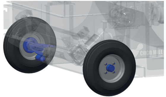
Grote rubberen wielen voor onverhard terrein Large rubber wheels for unpaved terrain Grandes ruedas de goma para uso todoterreno
